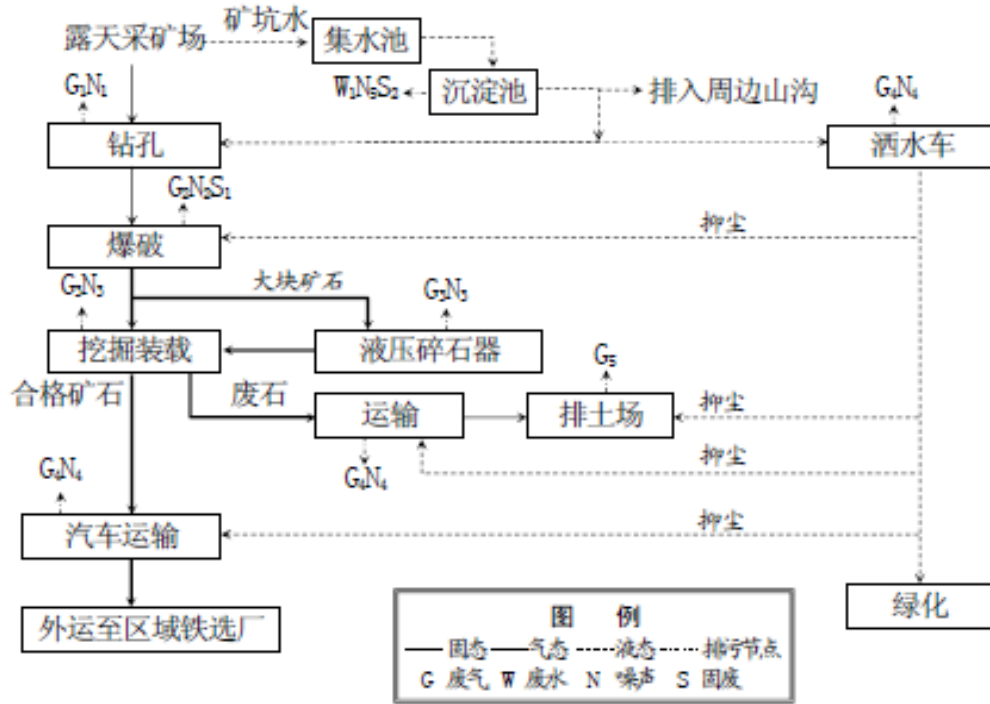
图 4-1 生产工艺流程图及排污节点
